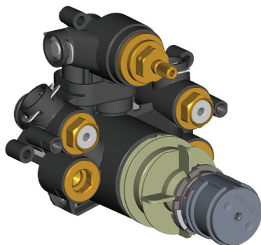
Термостатен смесител Надежден термостатен затварящ механизъм, стоп-ventили, възвратен клапан и DICHT-FIX система.
