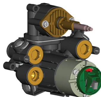
Едноръкохватков смесител Изберете вана/душ или смесител за душ с CLICK затварящ механизъм с функция за ограничение на температурата и водоспестяваща ECO функция и DICHT-FIX система.
